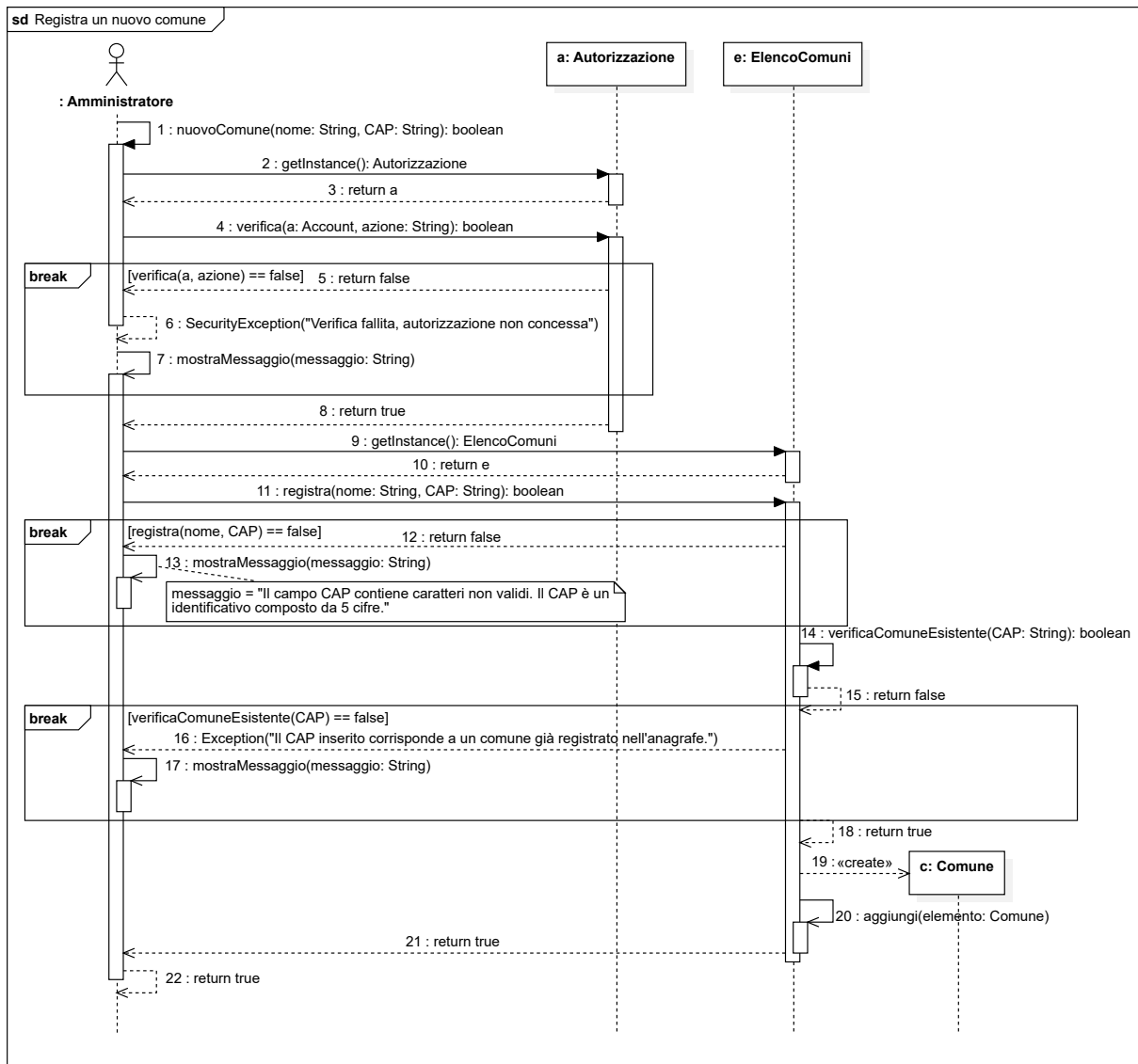
Diagramma delle sequenze 7: Registra un nuovo comune.
